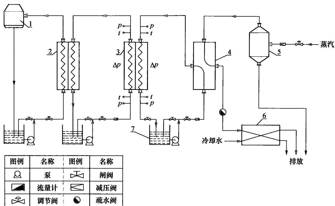
1—冷却塔, 2—冷却器, 3—热交换器试件, 4—加热器, 5—分离器, 6—过热器, 7—液体储槽, t —温度测口, p —压力测口
